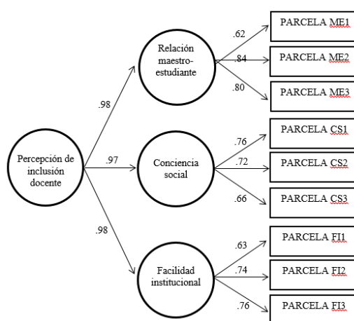
Figura 1. Modelo de covarianzas de la escala de percepción de inclusión docente. \chi^2=26.71 , (19 gl), p=.111 ; BNNFI=.98, BNNFI=.99, CFI=.99, RMSEA=.03
